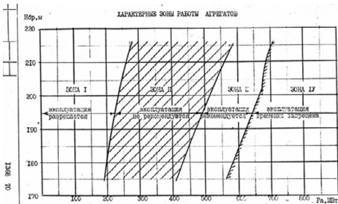
Рис.4.5.1. Эксплуатационная характеристика гидроагрегата с турбиной P0230/833-B-677
