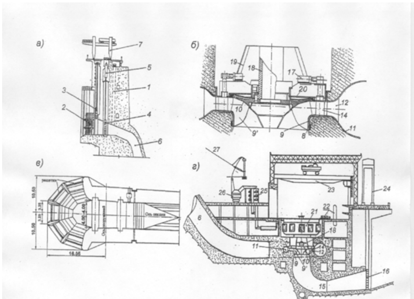
Рис.3.4 Турбинная установка с радиально-осевой турбиной Саяно-Шушенской ГЭС а) водоприемник; б) рабочее колесо; в) сороудерживающая решетка; г) здание ГЭС с водоводом, спиральной камерой, агрегатом и отсасывающей трубой.
